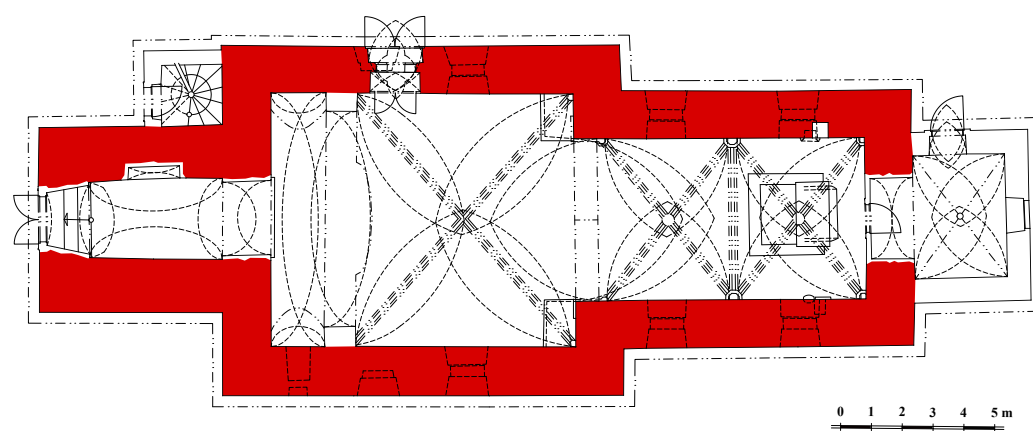
Vysoký Újezd, kostel Narození Panny Marie, půdorys s vyznačením středověkého zdiva
