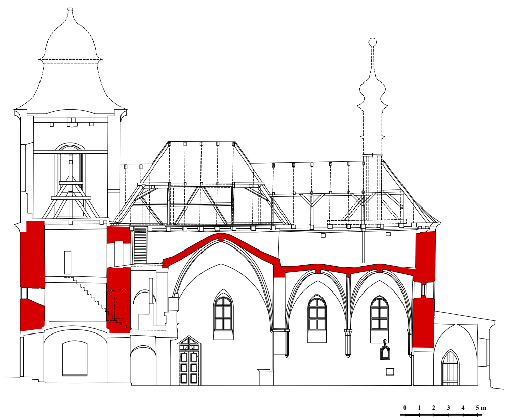
Vysoký Újezd, kostel NPM, podélný řez s vyznačením středověkých konstrukcí
