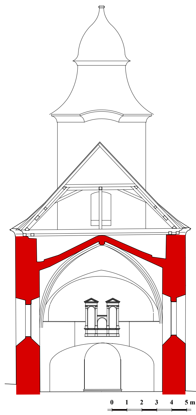
Vys. Újezd, kostel NPM, příčný řez s vyznačením středověkých konstrukcí
