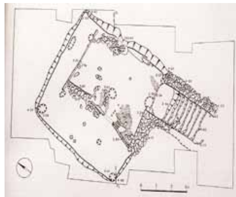
Půdorys objektu na Sekance, M. Richter.
