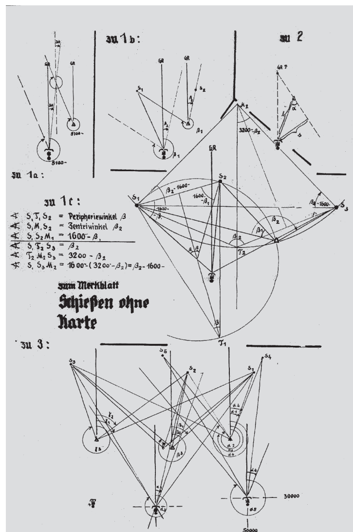
Výkres z dělostřelecké školy. Frekventanti škol absolvovali jak teoretický, tak praktický výcvik. Součástí dělostřelecké přípravy byly i výpočty trajektorií
