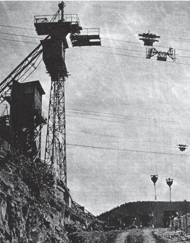
Lanovka spojující Teletínský lom se stavbou Slapské přehrady. Pamětníci vzpomínají, že i přes zákazy jezdili ve vozících z Teletína na Slapy a zpět. Musel to být hezký výhled.
